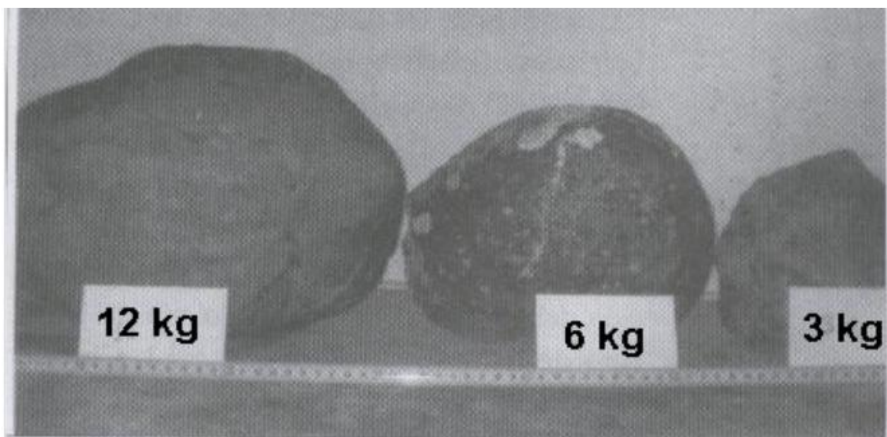
Fig. 11. Bolaños recogidos alrededor de la «Casa del Tolmillo»
